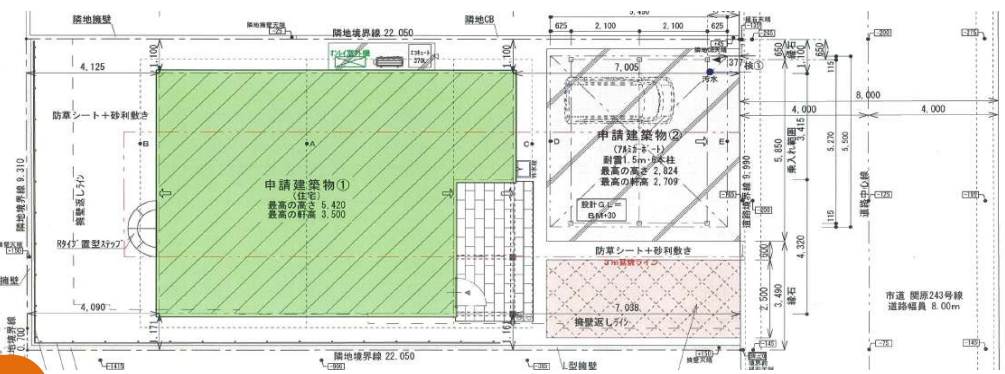
配置図
